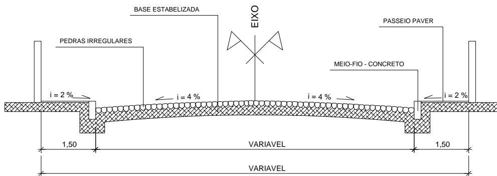
SECÇÃO TRANSVERSAL
