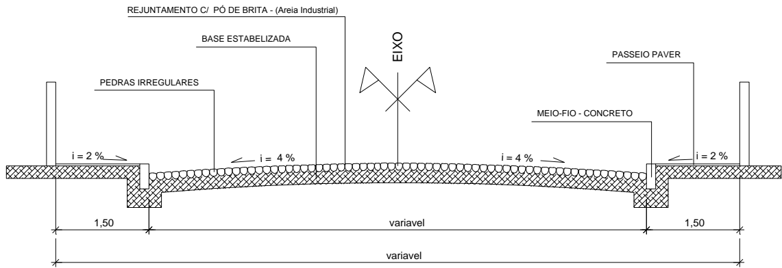
SECÇÃO TRANSVERSAL
