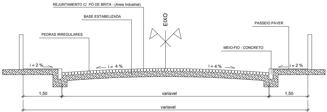
SECÇÃO TRANSVERSAL
