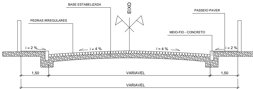
SECÇÃO TRANSVERSAL
